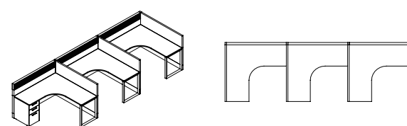
Vik66+vera42 F型3人工作站 4926*1666*1150mm
