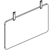
EFJ08 (木制挡板) W600 * D350 * H9 W800 * D350 * H9 W1000 * D350 * H9 W1200 * D350 * H9 W1400 * D350 * H9 W1600 * D350 * H9 W1800 * D350 * H9
