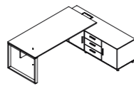
主管桌 DL88(L/R)-2 W2060*D1900*H750 W2260*D1900*H750
