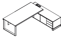
主管桌 DL89(L/R)-2 W2500*D2060*H750 W2300*D2060*H750
