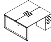
两人工位主桌 DL61-2.CG W1200*D1212*H750 W1400*D1412*H750 W1500*D1412*H750 W1600*D1412*H750
