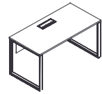
单人职员位主桌 DL60-2.GJ W1200*D600*H750 W1400*D700*H750 W1500*D700*H750 W1600*D700*H750
