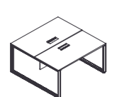
两人工位主桌 DL61-2.GJ W1200*D1212*H750 W1400*D1412*H750 W1500*D1412*H750 W1600*D1412*H750
