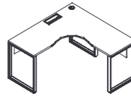
单人工位主桌 DL65(L/R)-2.GJ W1400*D1400*H750 W1500*D1500*H750 W1600*D1600*H750
