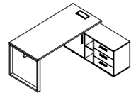
主管桌 DL86(L/R)-2 W1600*D1600*H750 W1800*D1600*H750
