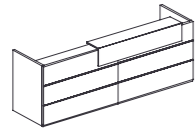
前台 DL81(L/R)-2 W2886*D841*H1126
