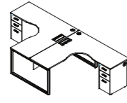
两人L工位主桌 DL62-2.CG W1400*D2812*H750 W1500*D3012*H750 W1600*D3212*H750
