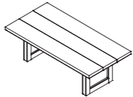
会议桌 EF78 Meeting Table W2400*D1200*H760
