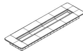
会议桌 EM78-2 W10000*D2800*H760
