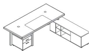
主台 EM85H-2 / EM85Z-2 W2400*D1050*H760 W2000*D1000*H760 W1800*D900*H760
