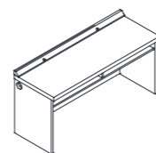
主席台 EM72-2 W800*D800*H760 W1400*D800*H760 W1600*D800*H760 W1800*D800*H760 W2000*D800*H760
