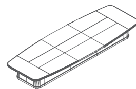
会议桌 EM77-2 W4800*D2200*H760 W6400*D2300*H760 W8000*D2370*H760
