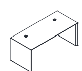
独立桌 EU21 Executive Desk W1800*D800*H760 W1600*D800*H760 W1400*D700*H760
