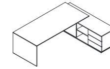
标准型主管桌 EU87 Executive Desk W2480*D1900*H760 W2280*D1900*H760 W2080*D1900*H760
