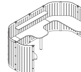
DY62.34 3420*1710*1400 DY62.34ZE 3362*1675*25
