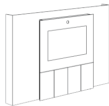
EI90 多媒体柜 Multimedia cabinet 3600(W)*448(D)*2360(H)
